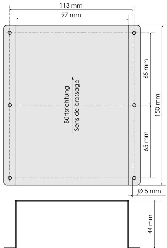
Massbild: RB150
