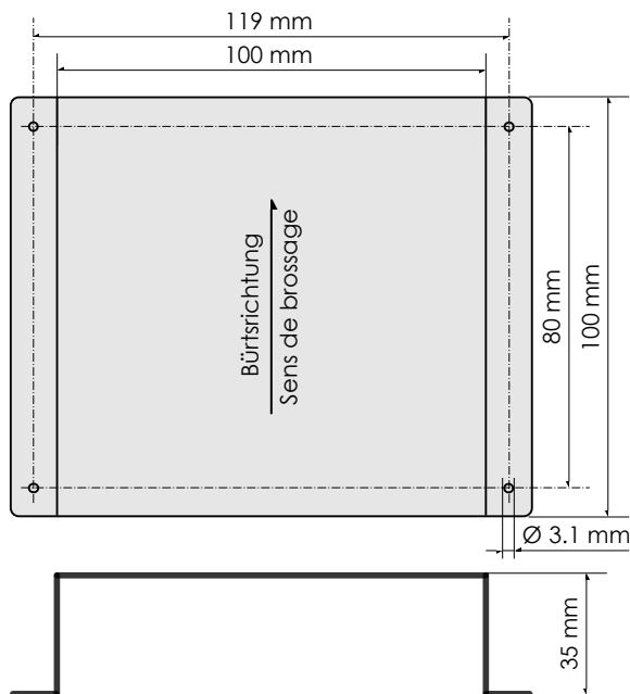
Massbild: RB100
