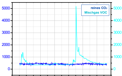
Anwendung in einer Toilette. Während der CO 2 -Sensor „gute“ Luft signalisiert, weiß es der VOC Mischgas-Sensor besser.
